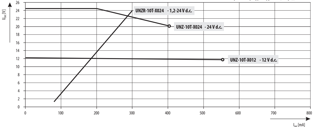
Нагрузочная характеристика UNZ-10T..., UNZR-10T-X024 - DC вывод
